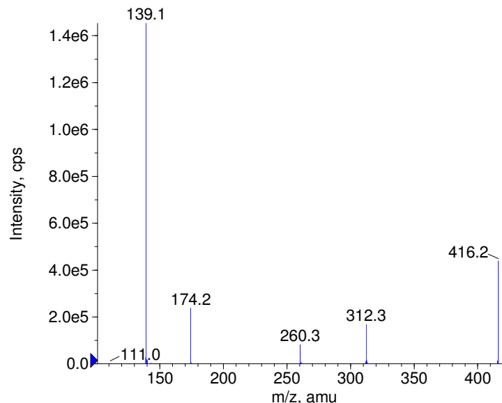
■ + Acemetacin Prec(416.0) CE(50.0) RT(0.5)
