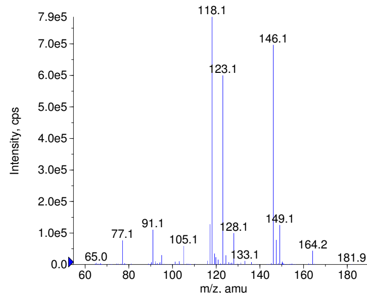
■ + Adrenalone Prec(182.0) CE(99.0) RT(0.9)
