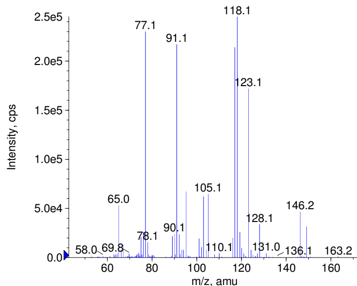
■ + Adrenalone Prec(182.0) CE(50.0) RT(0.8)
