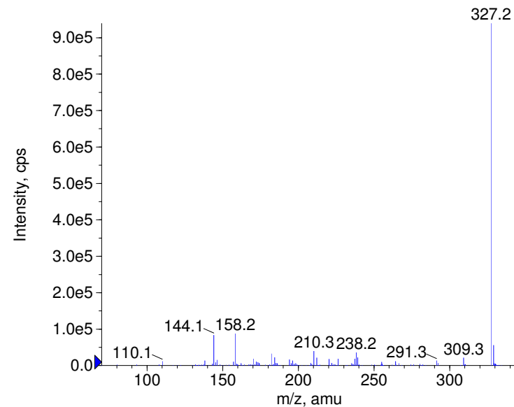
+ Ajmaline Prec(327.0) CE(99.0) RT(0.7)
