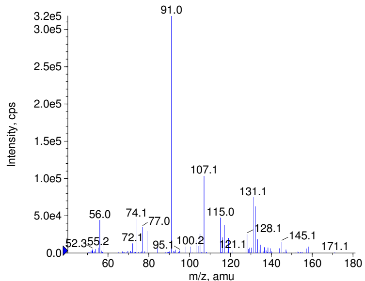
+ Alprenolol Prec(250.0) CE(50.0) RT(0.8)
