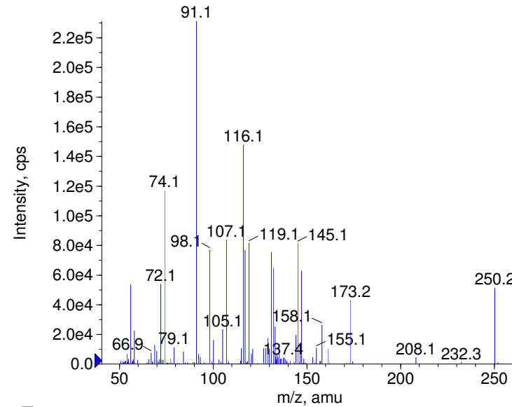
+ Alprenolol Prec(250.0) CE(99.0) RT(0.8)
