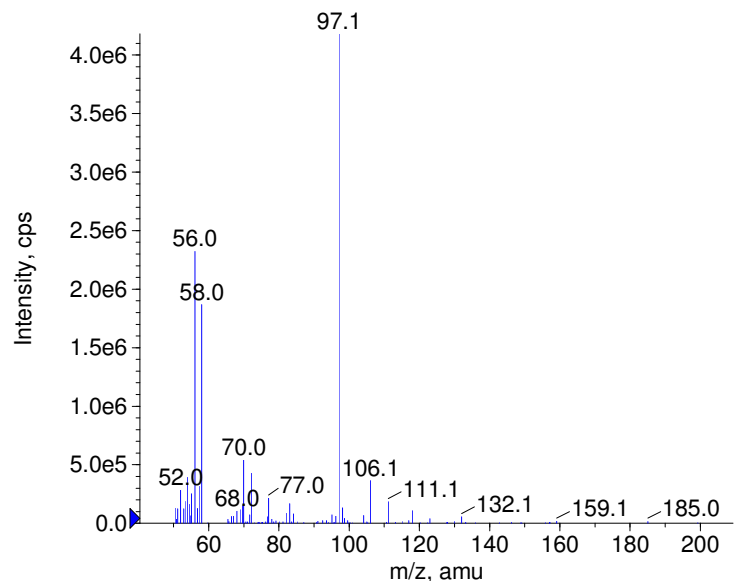
+ Amidopyrin Prec(232.0) CE(50.0) RT(1.0)
