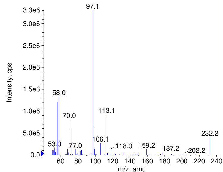
+ Amidopyrin Prec(232.0) CE(99.0) RT(1.0)
