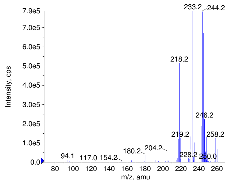
+ Azatadine Prec(291.0) CE(50.0) RT(0.8)
