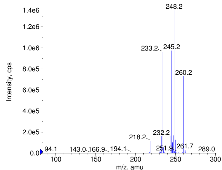
+ Azatadine Prec(291.0) CE(99.0) RT(0.8)
