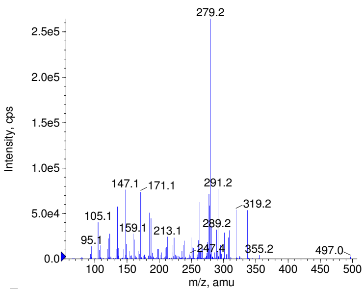
+ Betamethasone-17-benzoate Prec(497.0) CE(99.0) RT(1.6)
