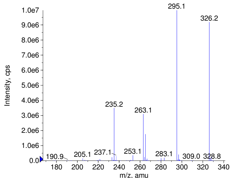
+ Bulbocapnin Prec(326.0) CE(50.0) RT(0.9)
