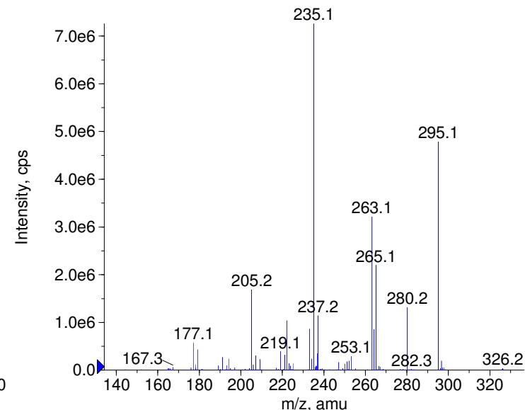
+ Bulbocapnin Prec(326.0) CE(99.0) RT(0.9)
