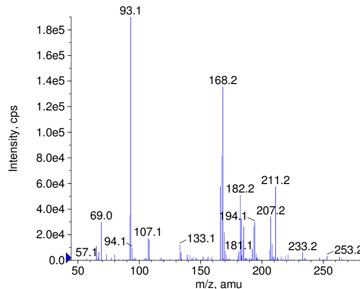
+ Bumadizone Prec(327.0) CE(50.0) RT(1.1)
