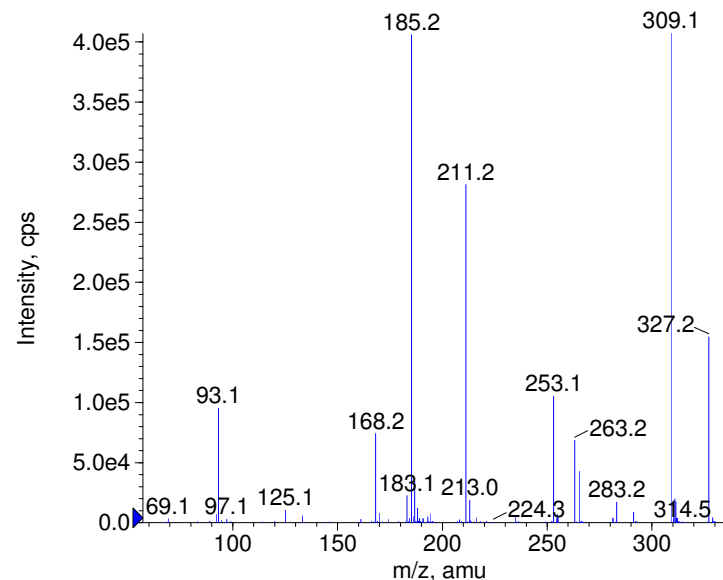
+ Bumadizone Prec(327.0) CE(50.0) RT(1.1)
