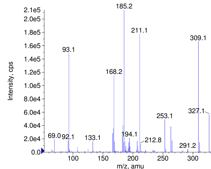
+ Bumadizone Prec(327.0) CE(99.0) RT(1.1)
