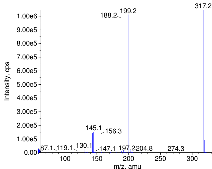
+ Butalamine Prec(317.0) CE(50.0) RT(0.9)
