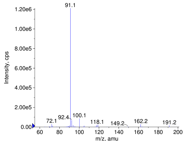
+ Butetamate Prec(264.0) CE(50.0) RT(0.9)
