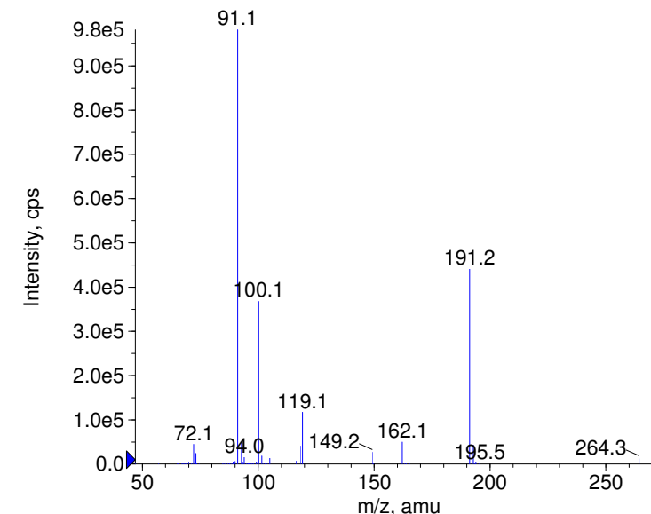
+ Butetamate Prec(264.0) CE(99.0) RT(0.9)
