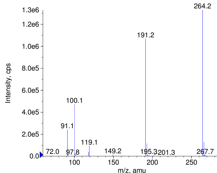
+ Butetamate Prec(264.0) CE(50.0) RT(0.9)
