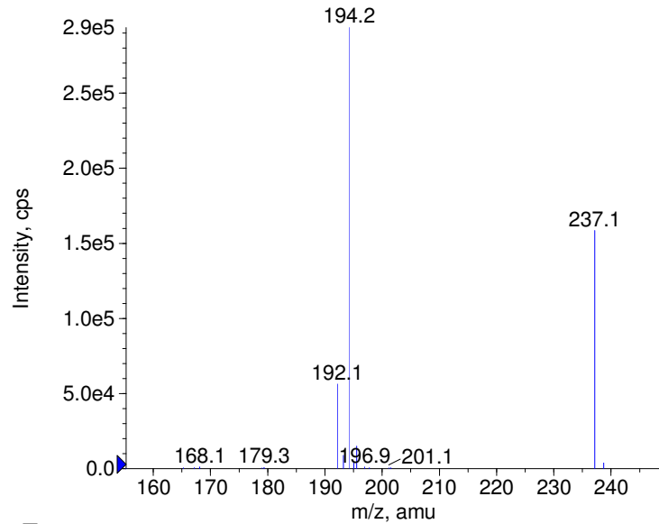
■ + Carbamazepine Prec(237.0) CE(50.0) RT(0.8)
