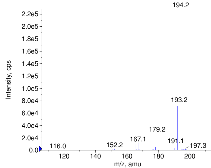
■ + Carbamazepine Prec(237.0) CE(99.0) RT(0.8)
