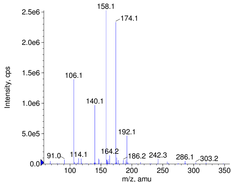
+ Cefalexin Prec(348.0) CE(50.0) RT(1.0)
