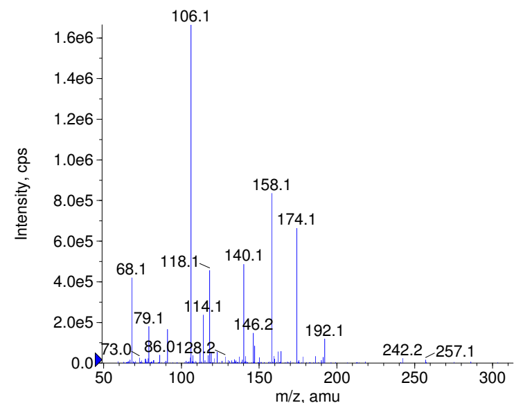
+ Cefalexin Prec(348.0) CE(99.0) RT(1.0)
