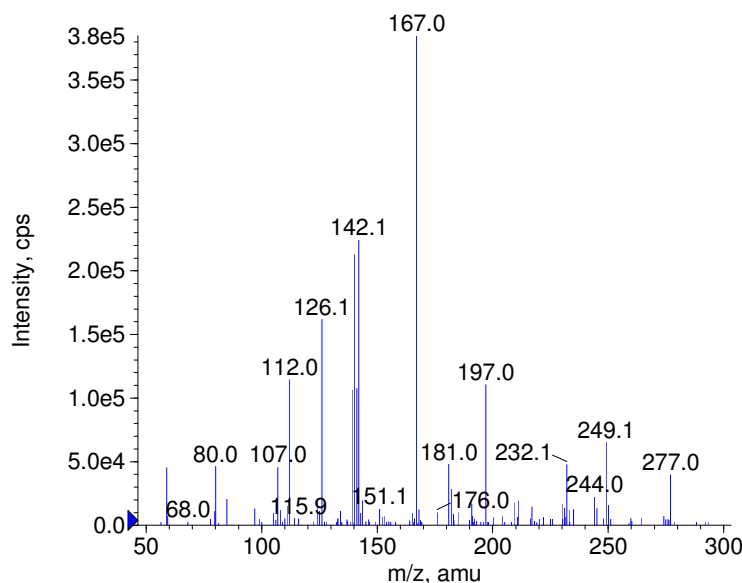
■ + Ceftazidime Prec(547.0) CE(50.0) RT(1.0)
