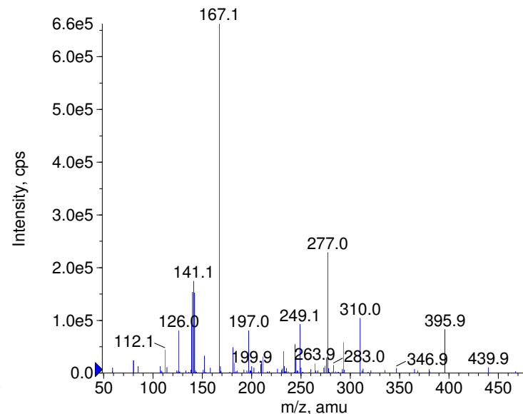
■ + Ceftazidime Prec(547.0) CE(99.0) RT(1.0)
