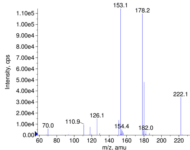
+ Chlorazaniil Prec(222.0) CE(99.0) RT(0.9)
