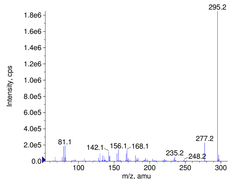
+ Cinchonidine Prec(295.0) CE(99.0) RT(1.0)
