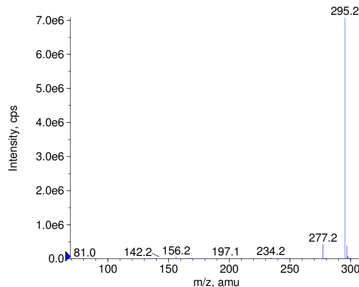
+ Cinchonidine Prec(295.0) CE(50.0) RT(1.0)
