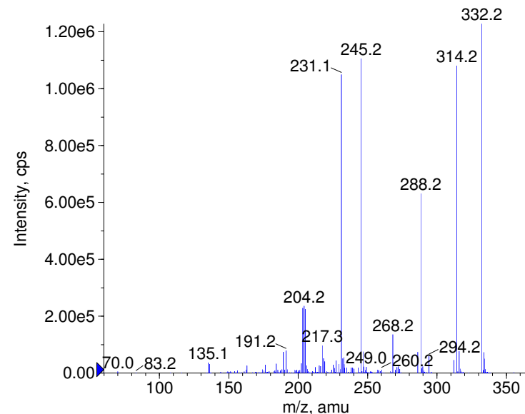
■ + Ciprofloxacin Prec(332.0) CE(99.0) RT(0.8)
