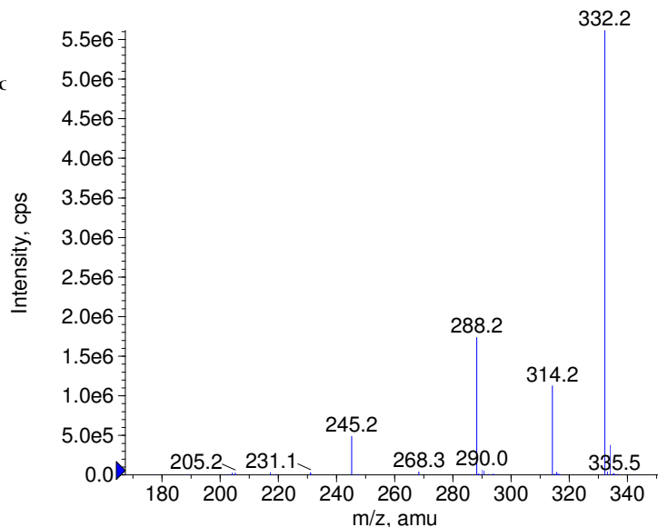
■ + Ciprofloxacin Prec(332.0) CE(50.0) RT(0.8)
