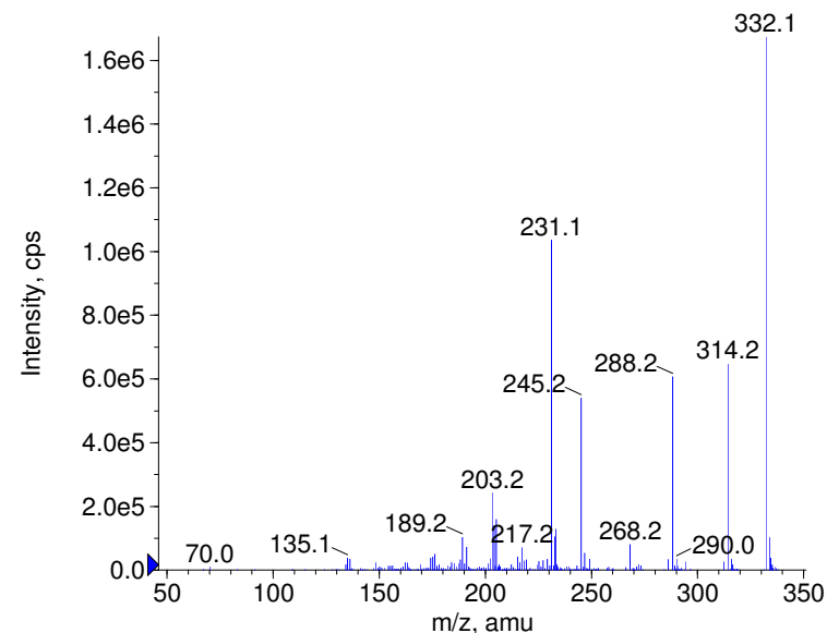
■ + Ciprofloxacin Prec(332.0) CE(99.0) RT(0.8)
