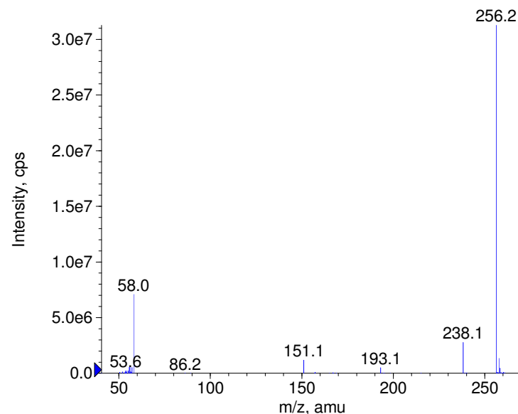
■ + Clobutinol Prec(256.0) CE(50.0) RT(0.8)
