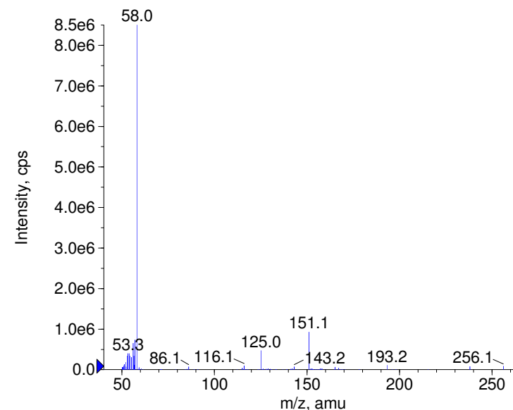
■ + Clobutinol Prec(256.0) CE(99.0) RT(0.9)
