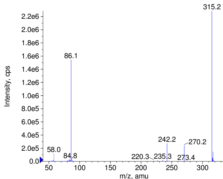
■ + Clomipramine Prec(315.0) CE(50.0) RT(0.8)
