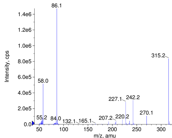
■ + Clomipramine Prec(315.0) CE(99.0) RT(0.8)
