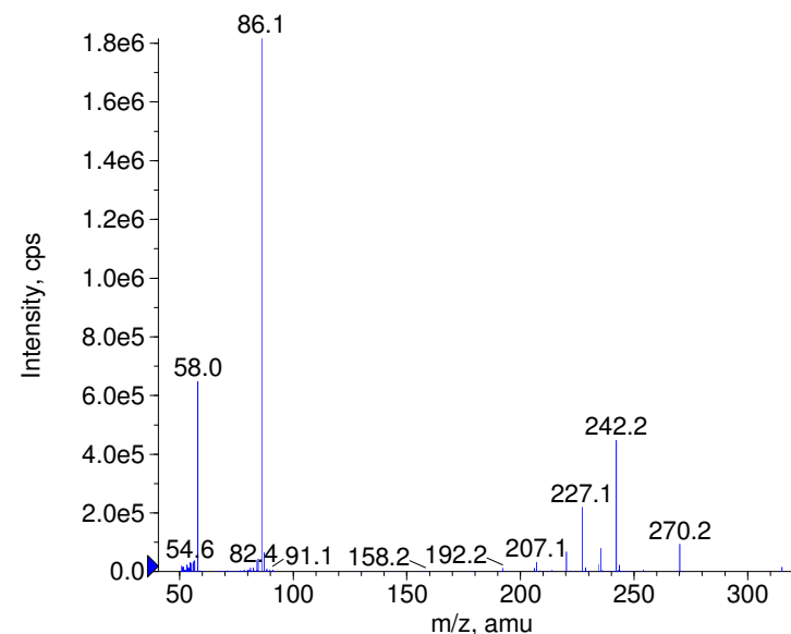
■ + Clomipramine Prec(315.0) CE(99.0) RT(0.8)
