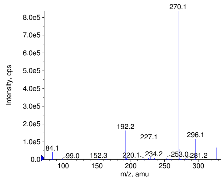
+ Clozapine Prec(327.0) CE(99.0) RT(0.8)
