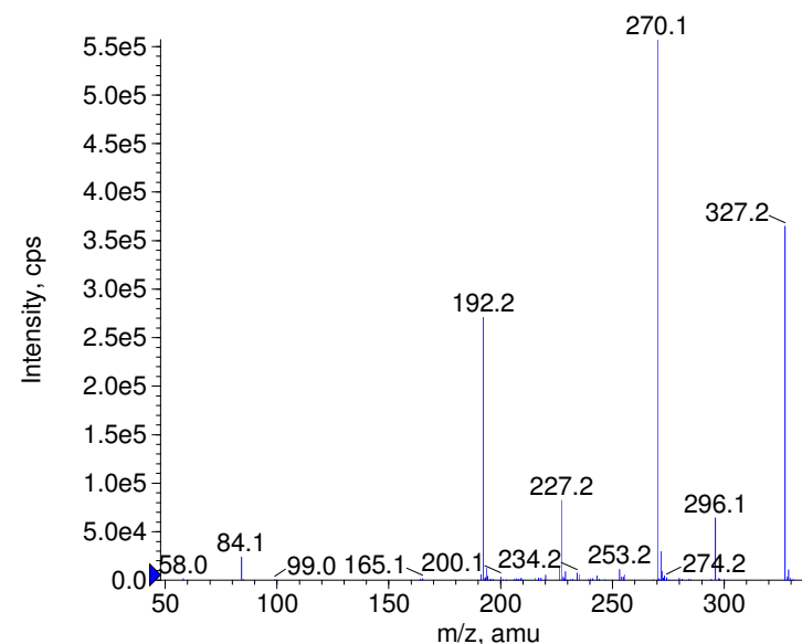
+ Clozapine Prec(327.0) CE(99.0) RT(0.8)
