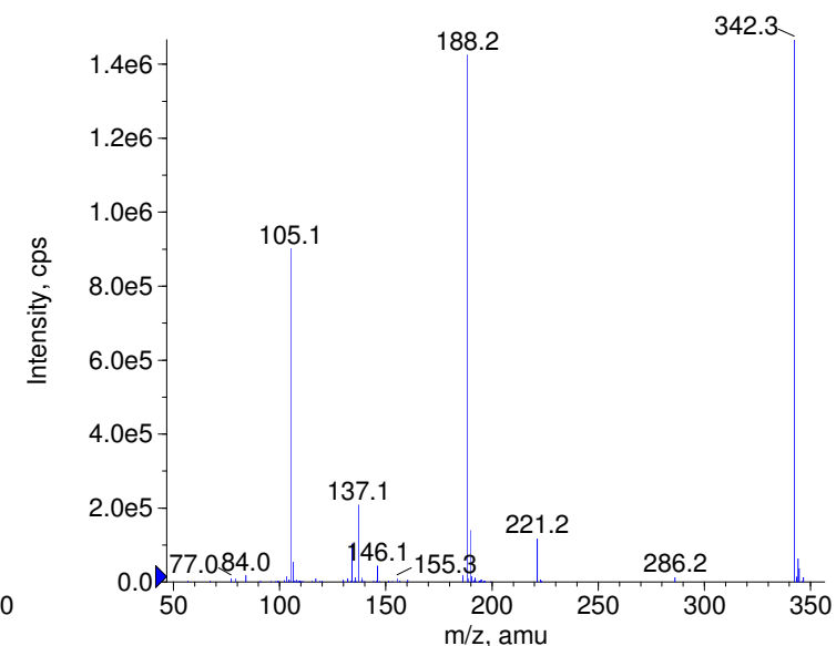
+ D5-Fentanyl Prec(342.0) CE(99.0) RT(0.8)
