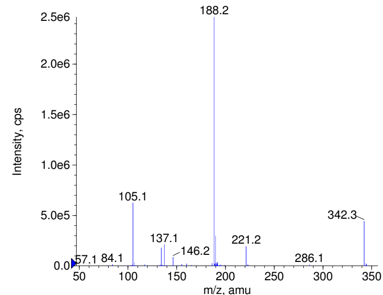
+ D5-Fentanyl Prec(342.0) CE(99.0) RT(0.8)
