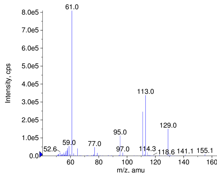
+ Demeton-O-methyl Prec(231.0) CE(50.0) RT(0.8)
