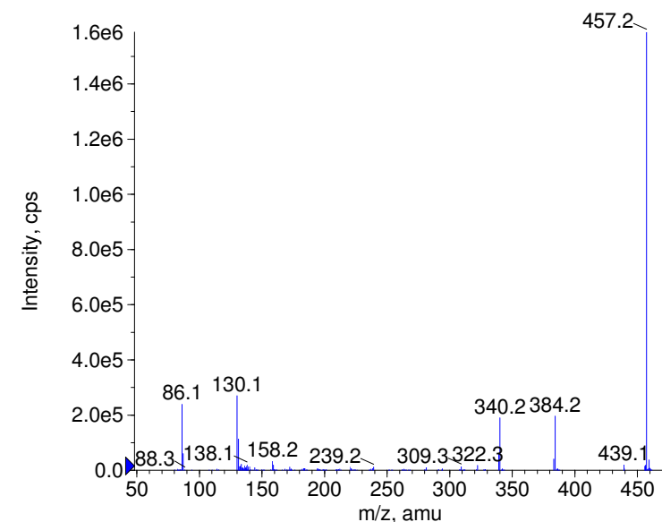
+ Detajmium Prec(457.0) CE(99.0) RT(1.1)
