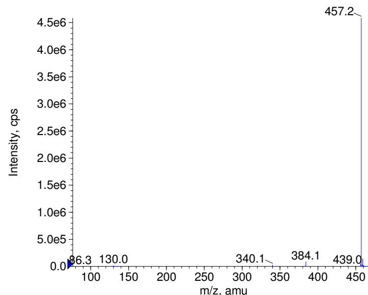
+ Detajmium Prec(457.0) CE(50.0) RT(1.1)
