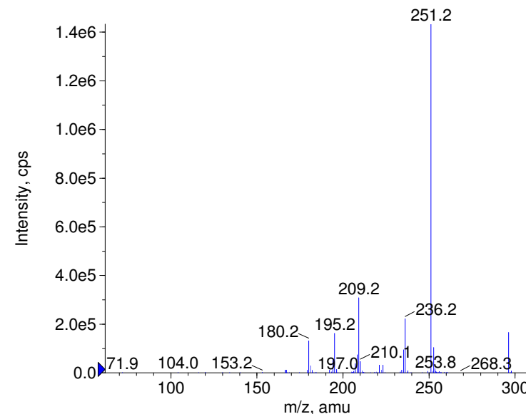
+ Dibenzepin Prec(296.0) CE(99.0) RT(0.7)
