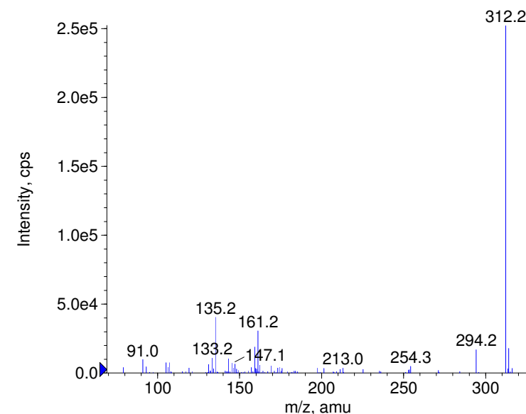
+ Dienogest Prec(312.0) CE(99.0) RT(0.9)
