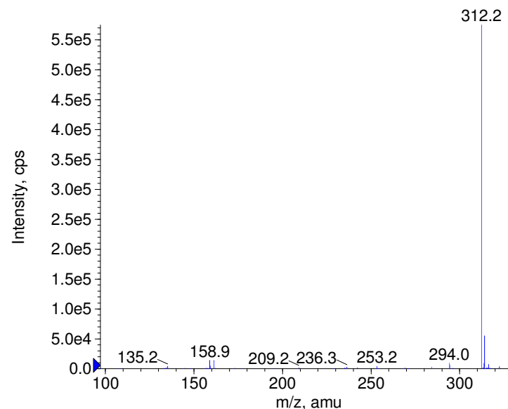
+ Dienogest Prec(312.0) CE(50.0) RT(0.9)
