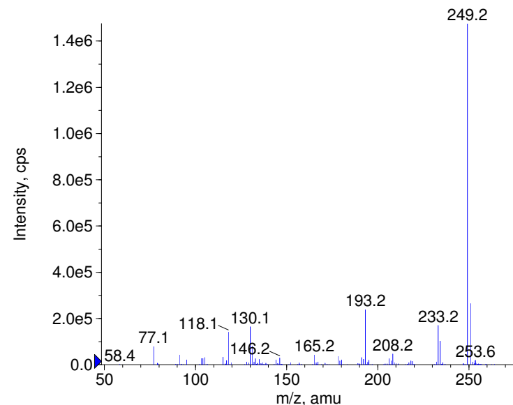
■ + Difenzoquat Prec(249.0) CE(99.0) RT(0.8)
