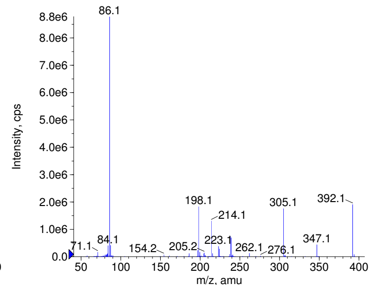
+ Dimetotiazine Prec(392.0) CE(99.0) RT(0.9)
