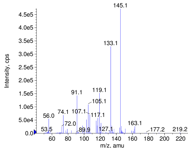
+ Esmolol Prec(296.0) CE(50.0) RT(0.9)
