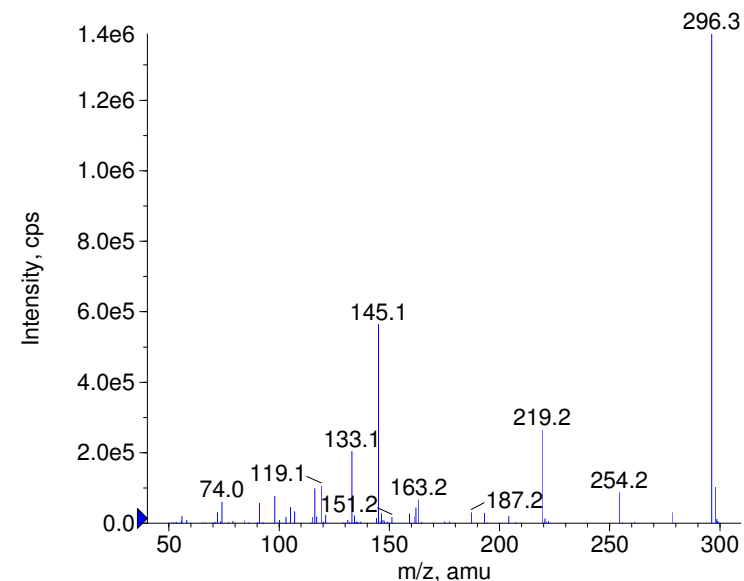
+ Esmolol Prec(296.0) CE(99.0) RT(0.9)
