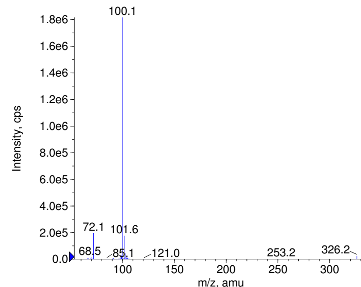
+ Etafenone Prec(326.0) CE(99.0) RT(0.9)
