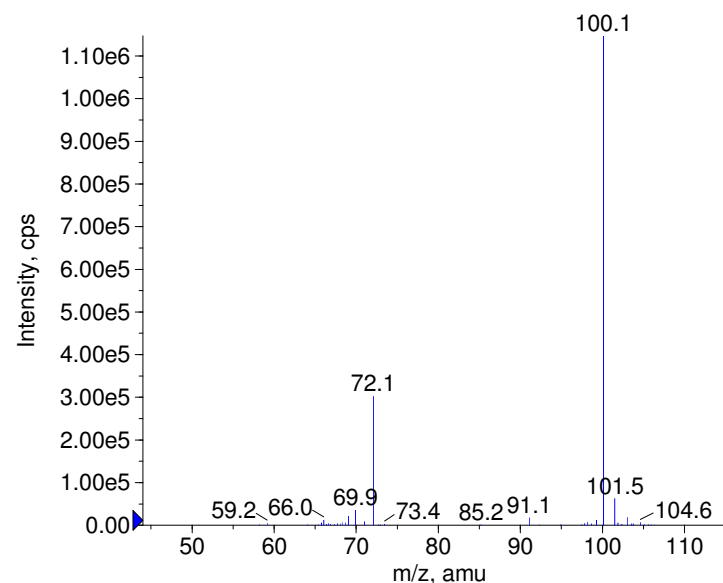
+ Etafenone Prec(326.0) CE(50.0) RT(0.8)
