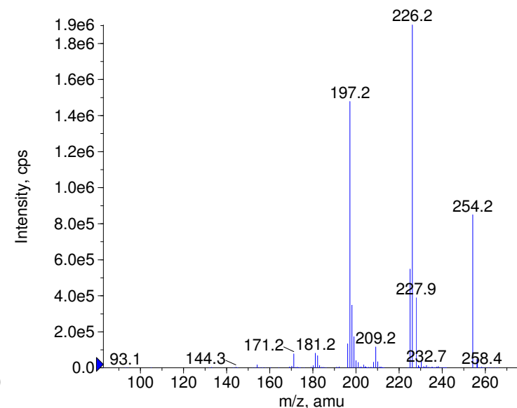
+ Ethacridine Prec(254.0) CE(99.0) RT(0.9)
