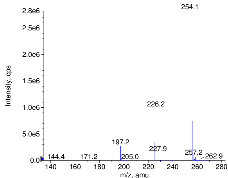
+ Ethacridine Prec(254.0) CE(50.0) RT(0.9)
