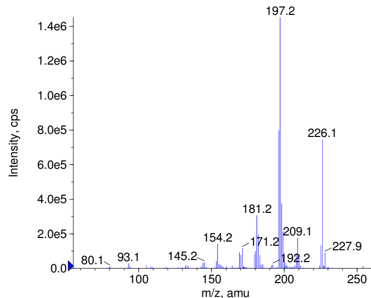
+ Ethacridine Prec(254.0) CE(50.0) RT(0.9)
