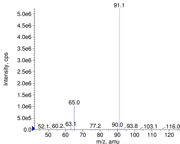
+ Etilamfetamine Prec(164.0) CE(50.0) RT(0.9)
