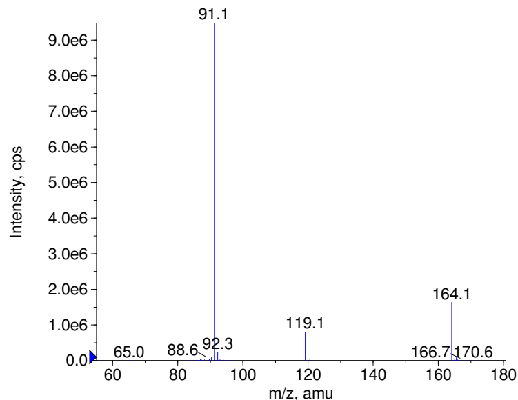
+ Etilamfetamine Prec(164.0) CE(50.0) RT(0.9)
