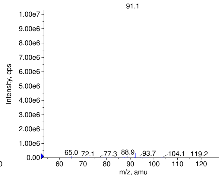
+ Etilamfetamine Prec(164.0) CE(99.0) RT(1.0)
