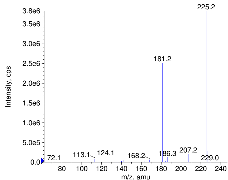
+ Etophylline Prec(225.0) CE(50.0) RT(0.8)
