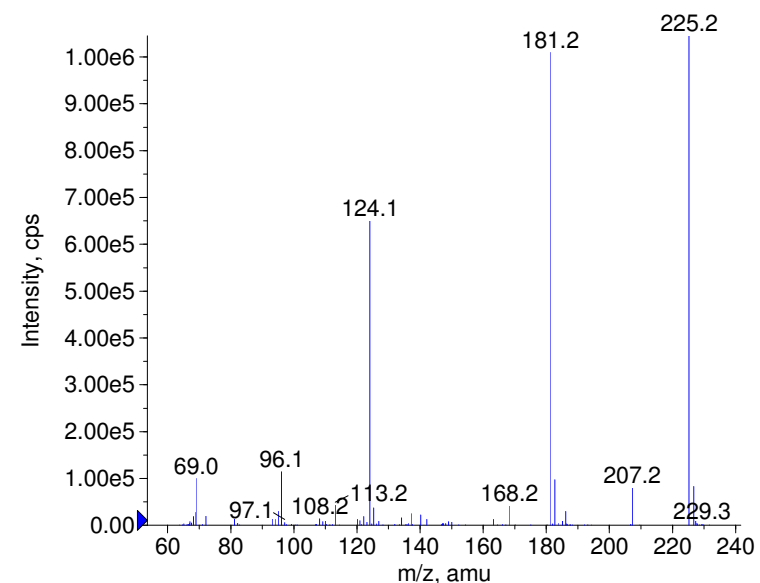
+ Etophylline Prec(225.0) CE(99.0) RT(0.9)
