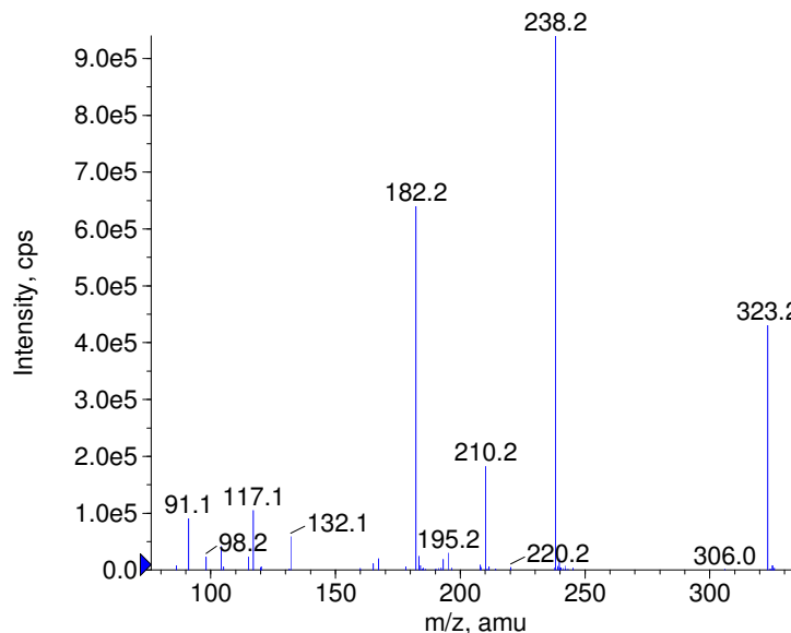
■ + Fenpipramide Prec(323.0) CE(99.0) RT(1.0)
