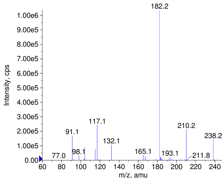
■ + Fenpipramide Prec(323.0) CE(50.0) RT(0.9)
