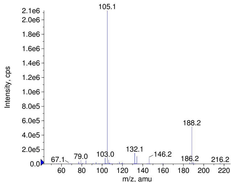
+ Fentanyl Prec(337.0) CE(50.0) RT(1.1)
