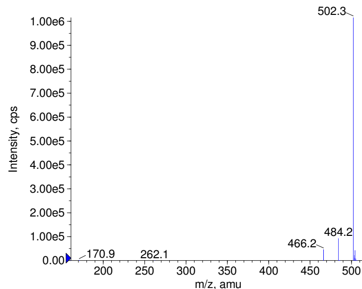
+ Fexofenadine Prec(502.0) CE(50.0) RT(0.7)
