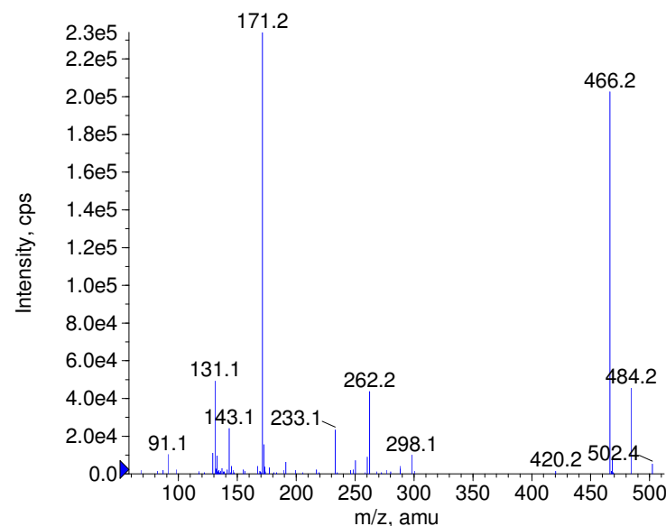
+ Fexofenadine Prec(502.0) CE(50.0) RT(0.7)
