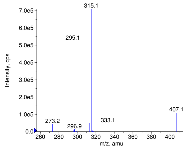
■ + Floctafenine Prec(407.0) CE(99.0) RT(1.0)
