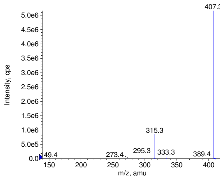
■ + Floctafenine Prec(407.0) CE(50.0) RT(1.0)
