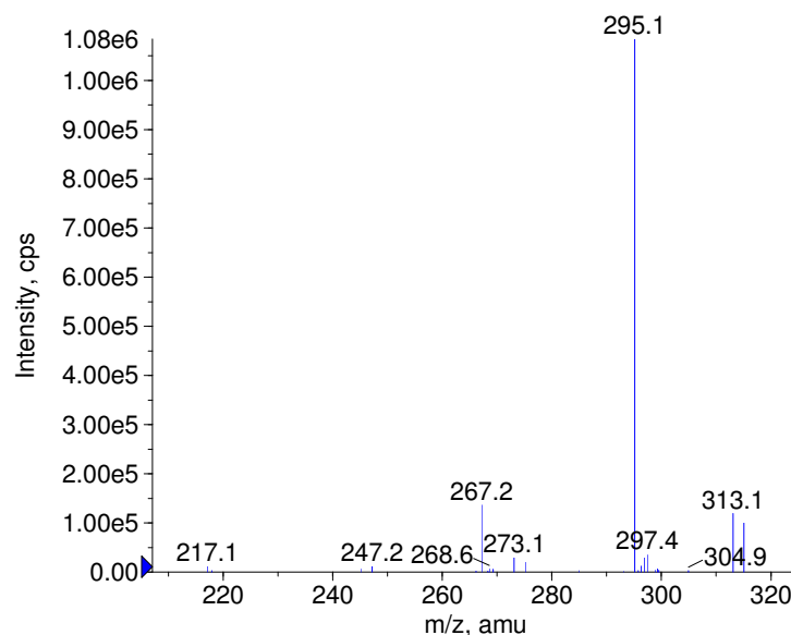
■ + Floctafenine Prec(407.0) CE(50.0) RT(1.0)
