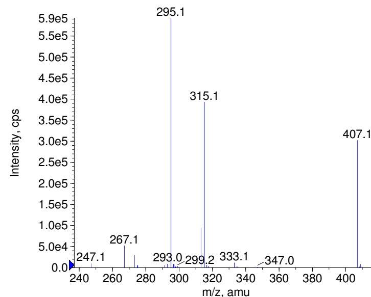
■ + Floctafenine Prec(407.0) CE(99.0) RT(1.0)
