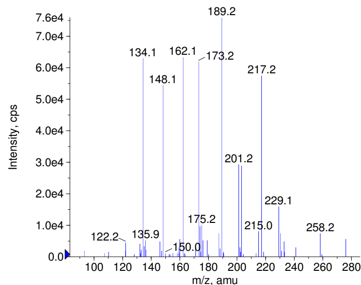
+ Flumazenil Prec(304.0) CE(50.0) RT(0.8)
