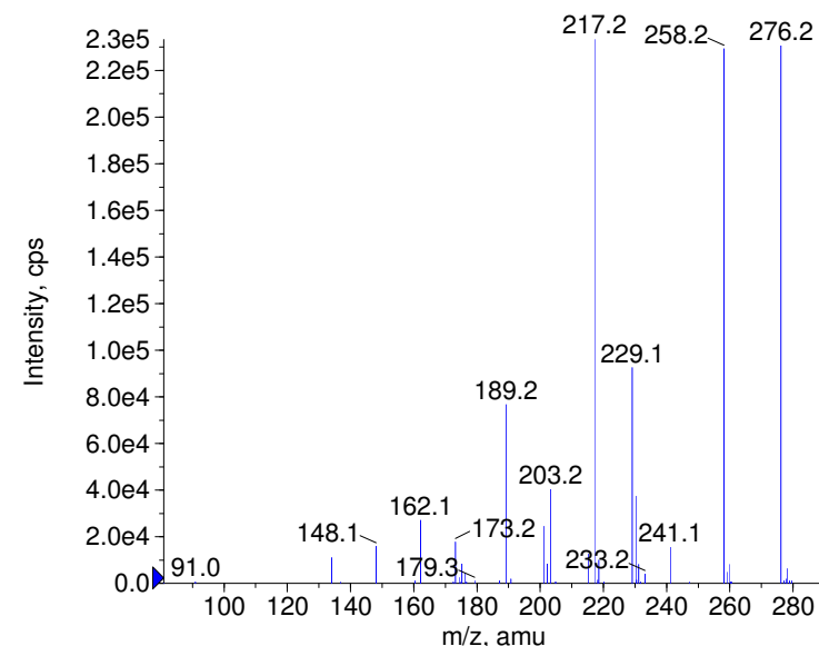
+ Flumazenil Prec(304.0) CE(99.0) RT(0.8)
