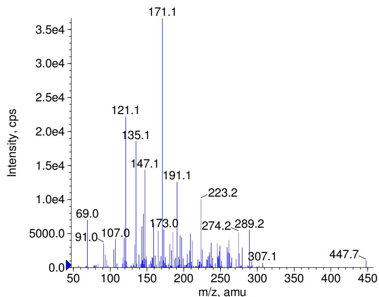
+ Fluocortin Butyl Prec(447.0) CE(50.0) RT(2.0)
