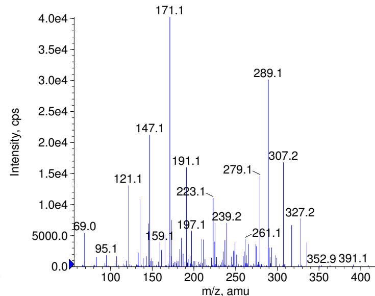
+ Fluocortin Butyl Prec(447.0) CE(99.0) RT(2.0)
