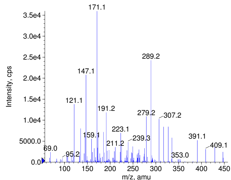
+ Fluocortin Butyl Prec(447.0) CE(99.0) RT(2.0)
