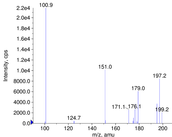
■ - Flurbiprofen Prec(243.0) CE(-50.0) RT(1.4)
