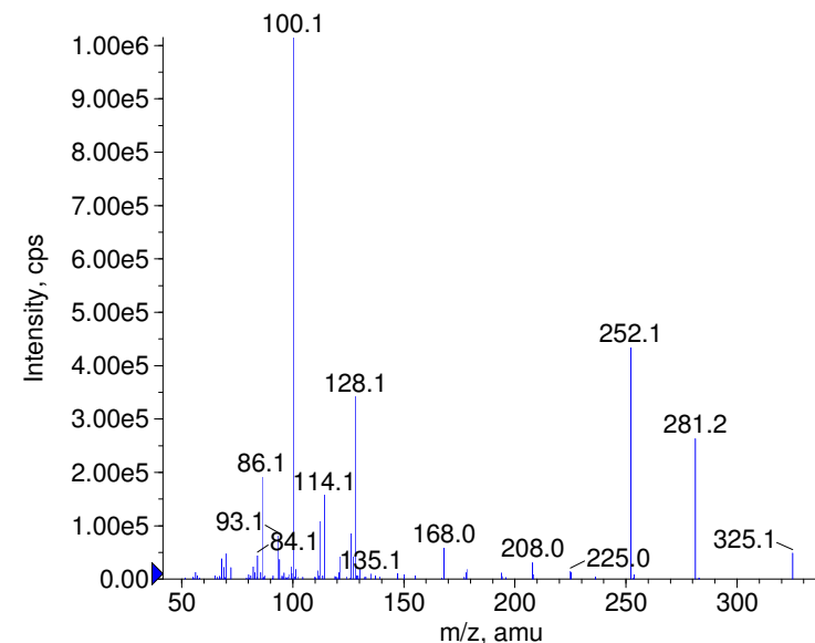
■ + Furaltadone Prec(325.0) CE(99.0) RT(1.0)
