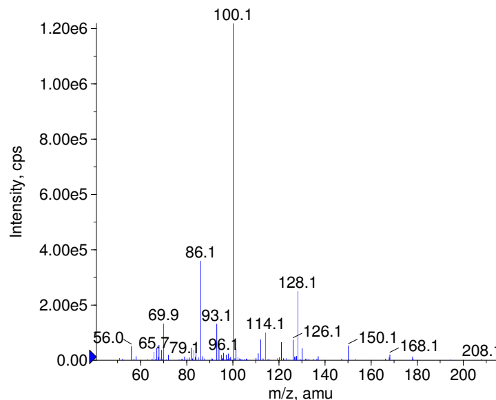
■ + Furaltadone Prec(325.0) CE(50.0) RT(0.9)
