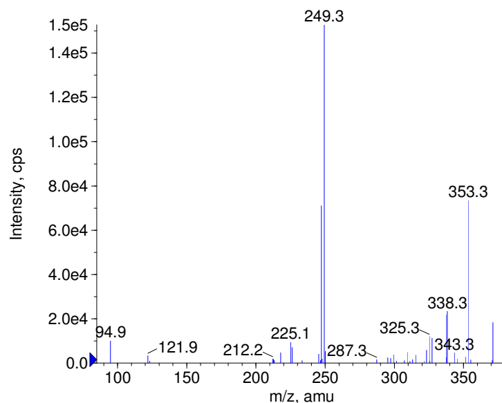
■ - Gitoxigenin Prec(389.0) CE(-50.0) RT(0.8)
