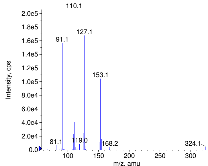
+ Gliclazide Prec(324.0) CE(99.0) RT(0.9)
