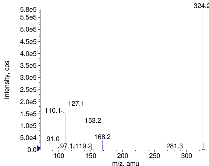
+ Gliclazide Prec(324.0) CE(50.0) RT(0.9)
