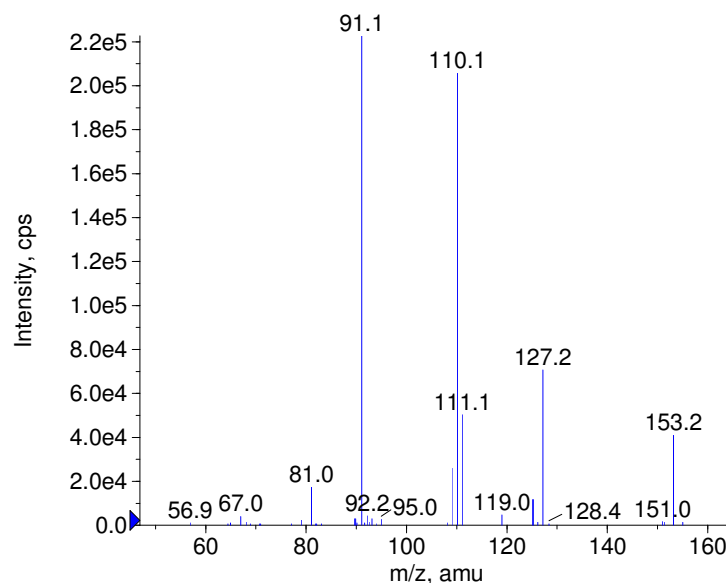
+ Gliclazide Prec(324.0) CE(50.0) RT(0.9)
