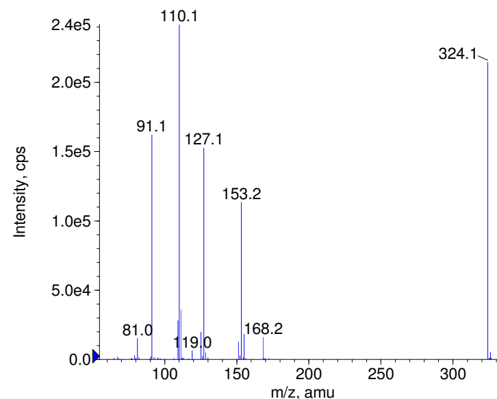
+ Gliclazide Prec(324.0) CE(99.0) RT(0.9)
