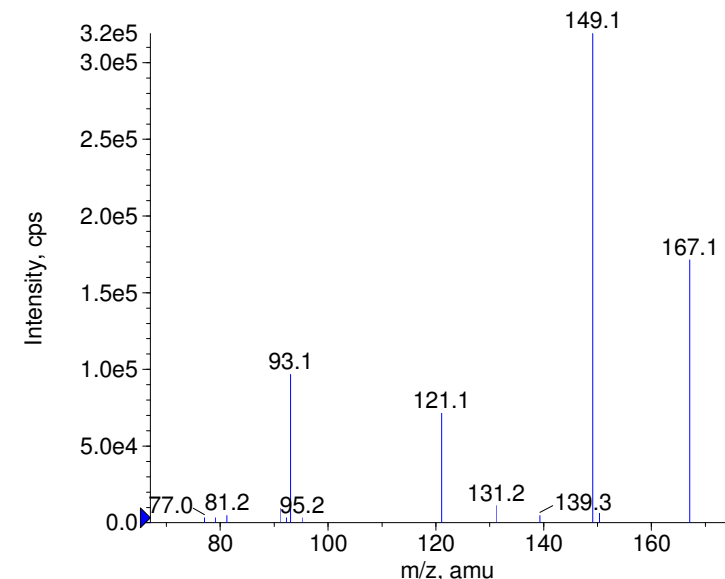
+ Hapargosid Prec(495.0) CE(99.0) RT(0.9)
