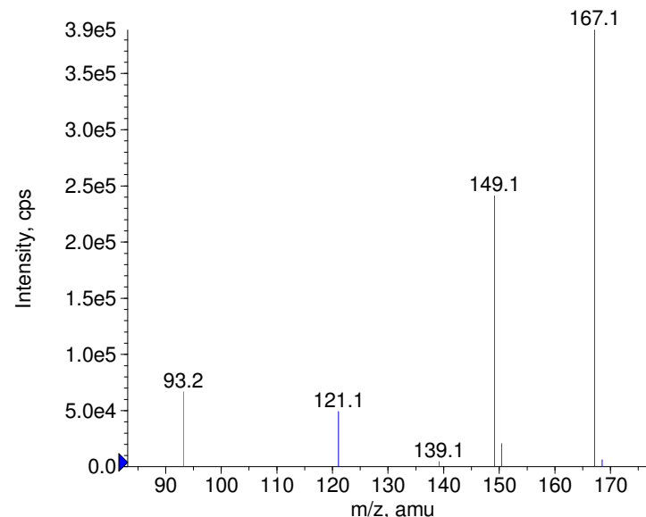
+ Hapargosid Prec(495.0) CE(50.0) RT(0.9)
