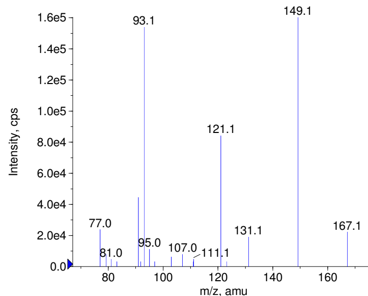
+ Hapargosid Prec(495.0) CE(50.0) RT(0.9)
