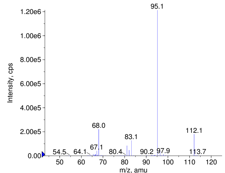
+ Histamine Prec(112.0) CE(99.0) RT(1.2)
