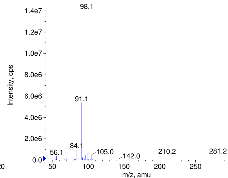
+ Histapyrrodine Prec(281.0) CE(99.0) RT(0.9)
