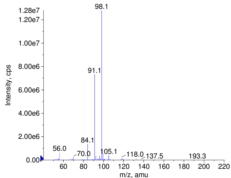
+ Histapyrrodine Prec(281.0) CE(50.0) RT(0.9)
