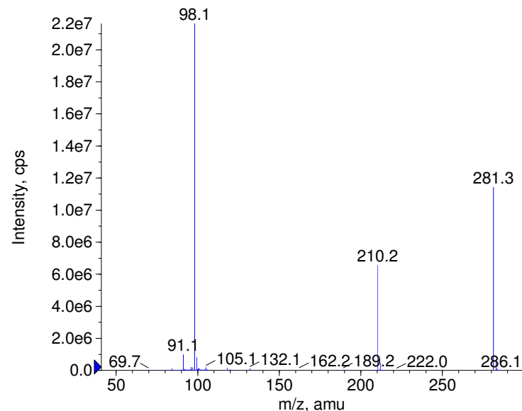
+ Histapyrrodine Prec(281.0) CE(50.0) RT(0.9)
