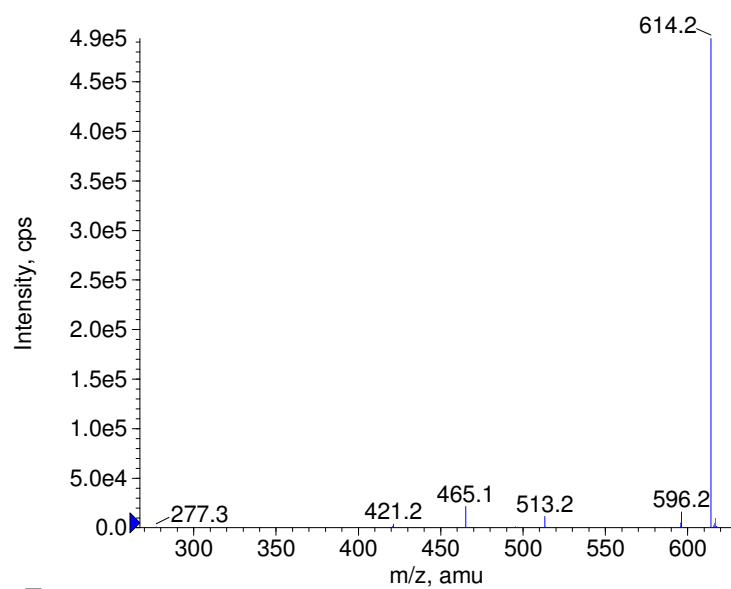
+ Indinavir Prec(614.0) CE(50.0) RT(0.8)
