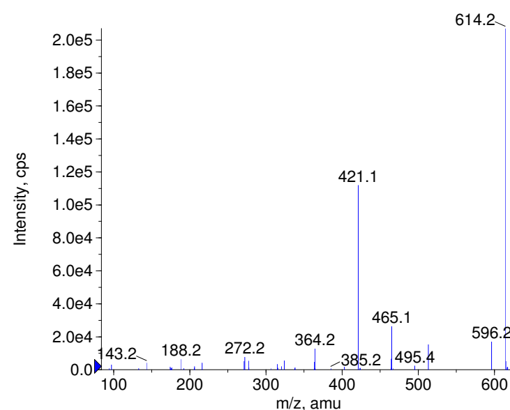
+ Indinavir Prec(614.0) CE(99.0) RT(0.8)
