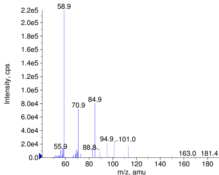
■ - Lactitol Prec(343.0) CE(-50.0) RT(0.9)
