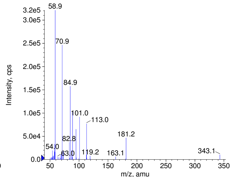
■ - Lactitol Prec(343.0) CE(-99.0) RT(0.9)
