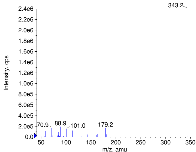
■ - Lactitol Prec(343.0) CE(-50.0) RT(0.9)
