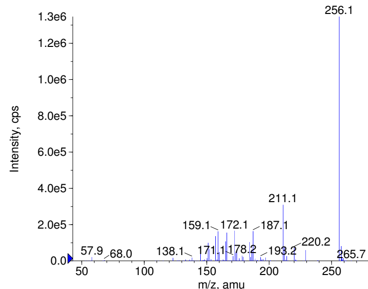
■ + Lamotrigine Prec(256.0) CE(99.0) RT(0.7)
