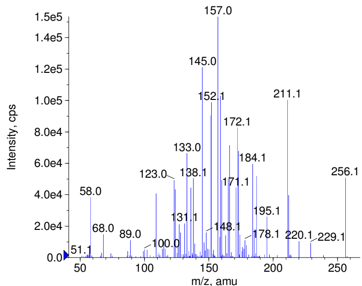
■ + Lamotrigine Prec(256.0) CE(50.0) RT(0.7)
