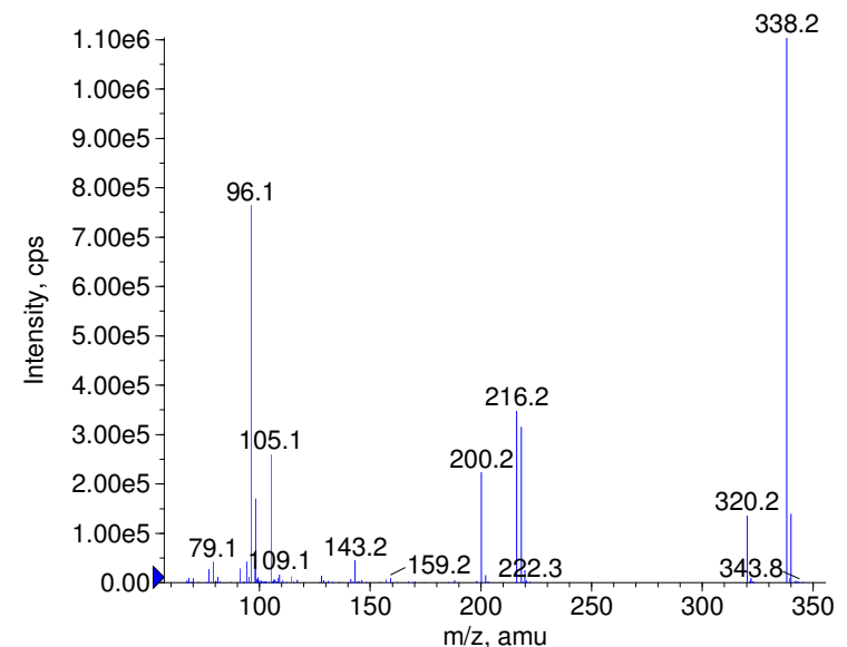
+ Lobeline Prec(338.0) CE(99.0) RT(0.9)
