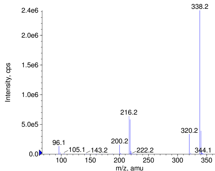
+ Lobeline Prec(338.0) CE(50.0) RT(0.8)
