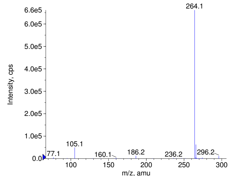
+ Mebendazole Prec(296.0) CE(99.0) RT(0.8)
