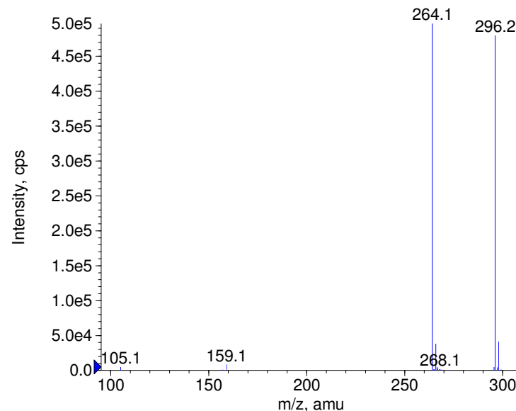
+ Mebendazole Prec(296.0) CE(50.0) RT(0.8)
